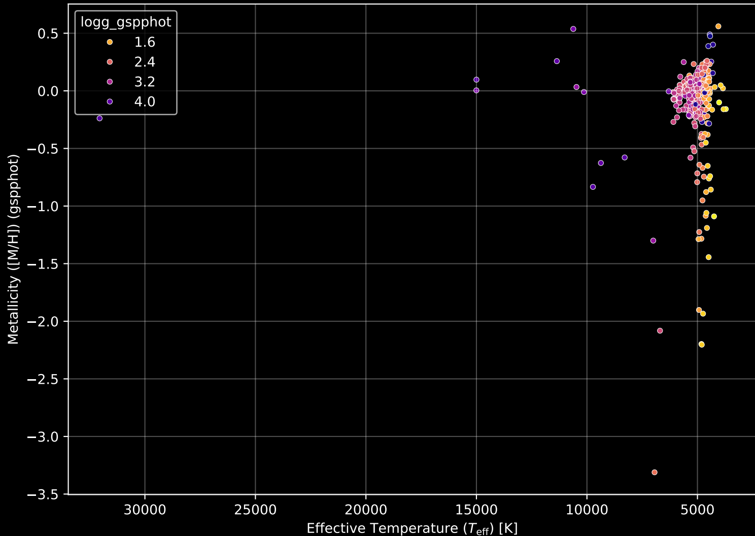
APOGEE DR17 Field: [146+08] Stellar Population Parameters (n= 333)
